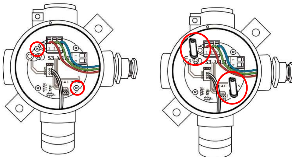
Sustituir tornillos por torretas
