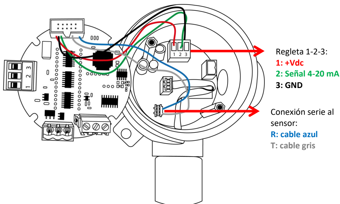
Conexión del módulo display al sensor remoto mediante conexión serie
