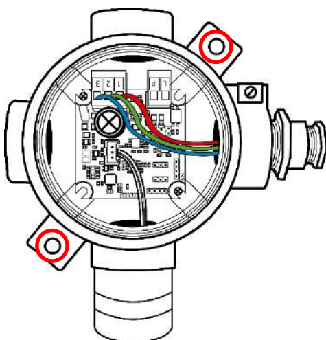
Figura 8: Instalación S/3-IR ATEX
