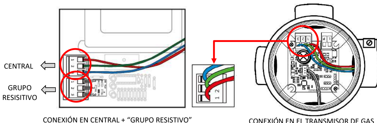
Figura 11: Conexión Central-Transmisor de gas
