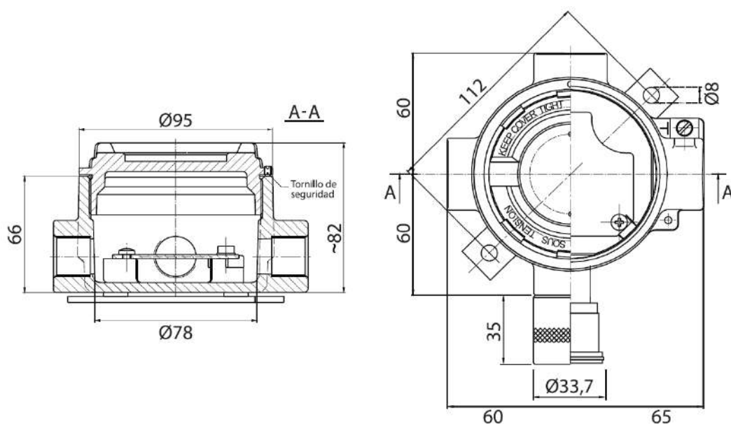
Figura 6: Planos y cota del transmisor de gas S/3-IR
