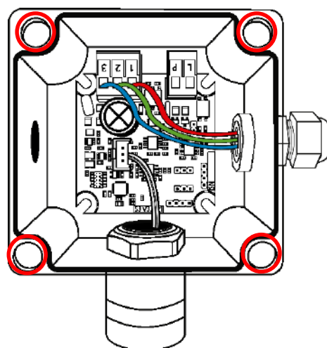
Figura 9: Instalación S/2-IR ABS
