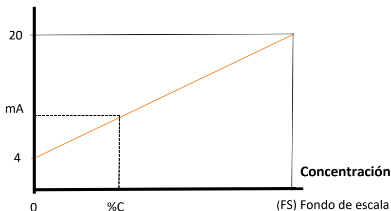
Salida 4-20 mA
