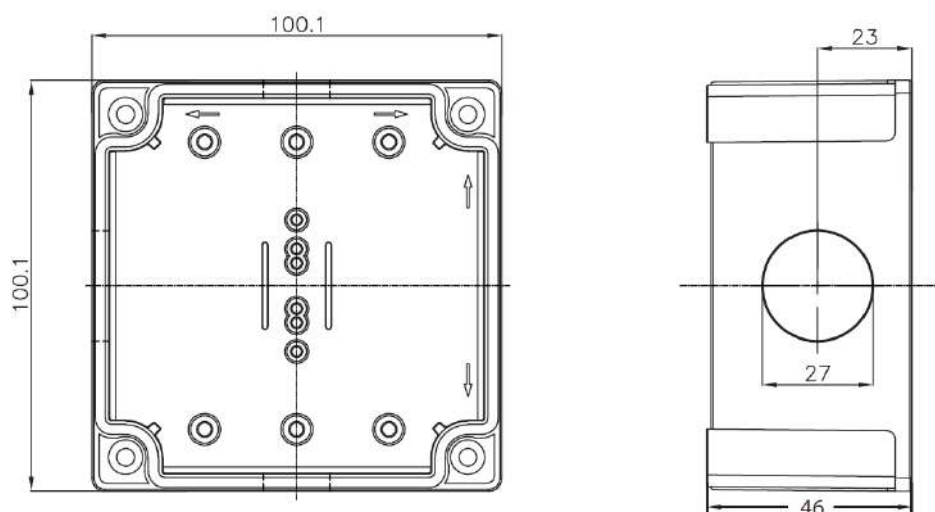
Figura 7: Planos y cotas del transmisor de gas S/2-IR
