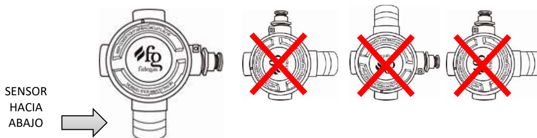
Figura 4: posición correcta de colocación del sensor Figura 5: posiciones incorrectas de colocación del sensor
