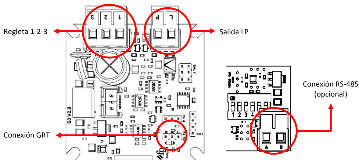
Figura 10: Conexiones
