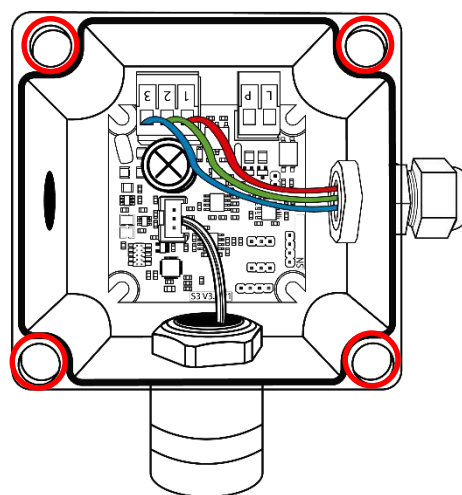
Figura 8: Instalación S/2-T2 ABS
