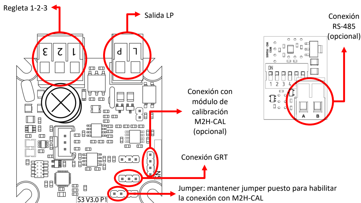
Figura 9: Conexiones
