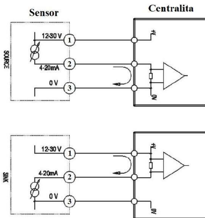
Figura 2. Configuración SINK y SOURCE
