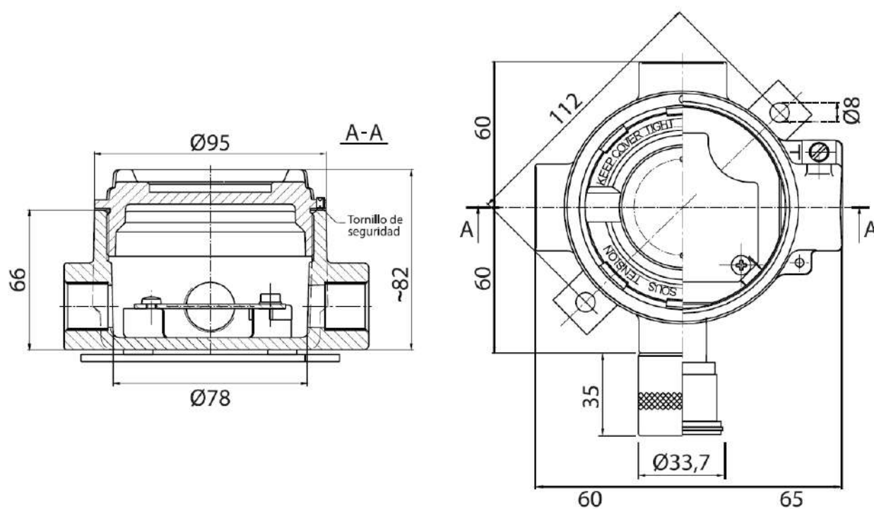
Figura 5: Planos y cotas del transmisor de gas S/3-T2
