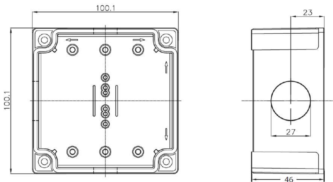
Figura 6: Planos y cotas del transmisor de gas S/2-T2
