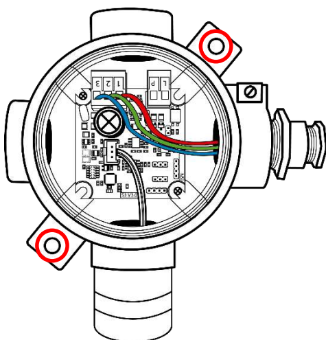
Figura 7: Instalación S/3-T2 ATEX
