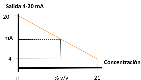
Figura 1: Relación entre la concentración y la salida 4-20 mA
